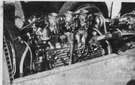
Arriba: Parte de la obra realizada en el país. El motor de serie con equipo de admisión especial alimentado por tres carburadores duales.
