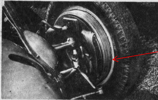
★ Otra de las riquezas de este chasis europeo. Los soberbios frenos amplios y muy bien ventilados y un brazo de dirección
