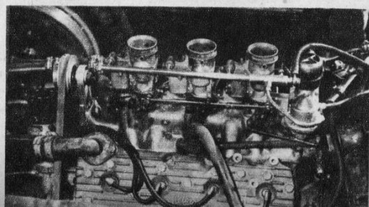
Arriba: Parte de la obra realizada en el país. El motor de serie con equipo de admisión especial alimentado por tres carburadores duales.
