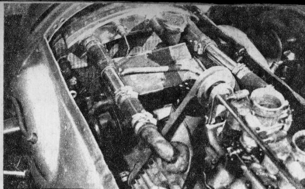
Los radiadores semidesnudos. El de agua más amplio, tiene tras sí al de lubricante viéndose el distribuidor y carburadores
